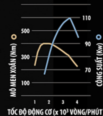
ĐỘNG CƠ 2GD - FTV 2.4L
