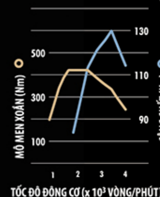
ĐỘNG CƠ 1GD - FTV 2.8L
